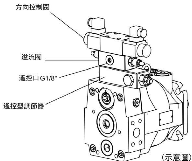
遙控型調節器+電控卸載+兩段壓力 GC
