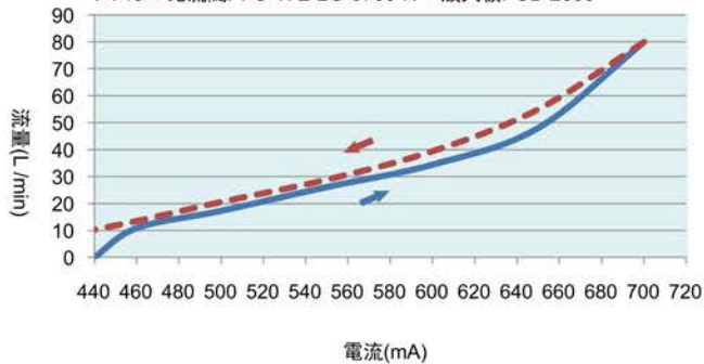
PV46 + 比流閥PFC-17E-2G-0700-N + 放大板PCB-2600
